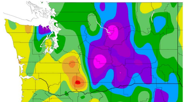
Temperature (°F)
